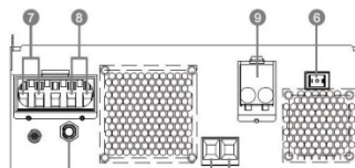
2кВт-3кВт одиночное исполнение
