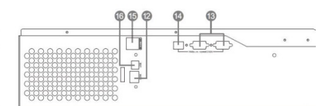
2кВт-5,5кВт исполнение для параллельной работы
